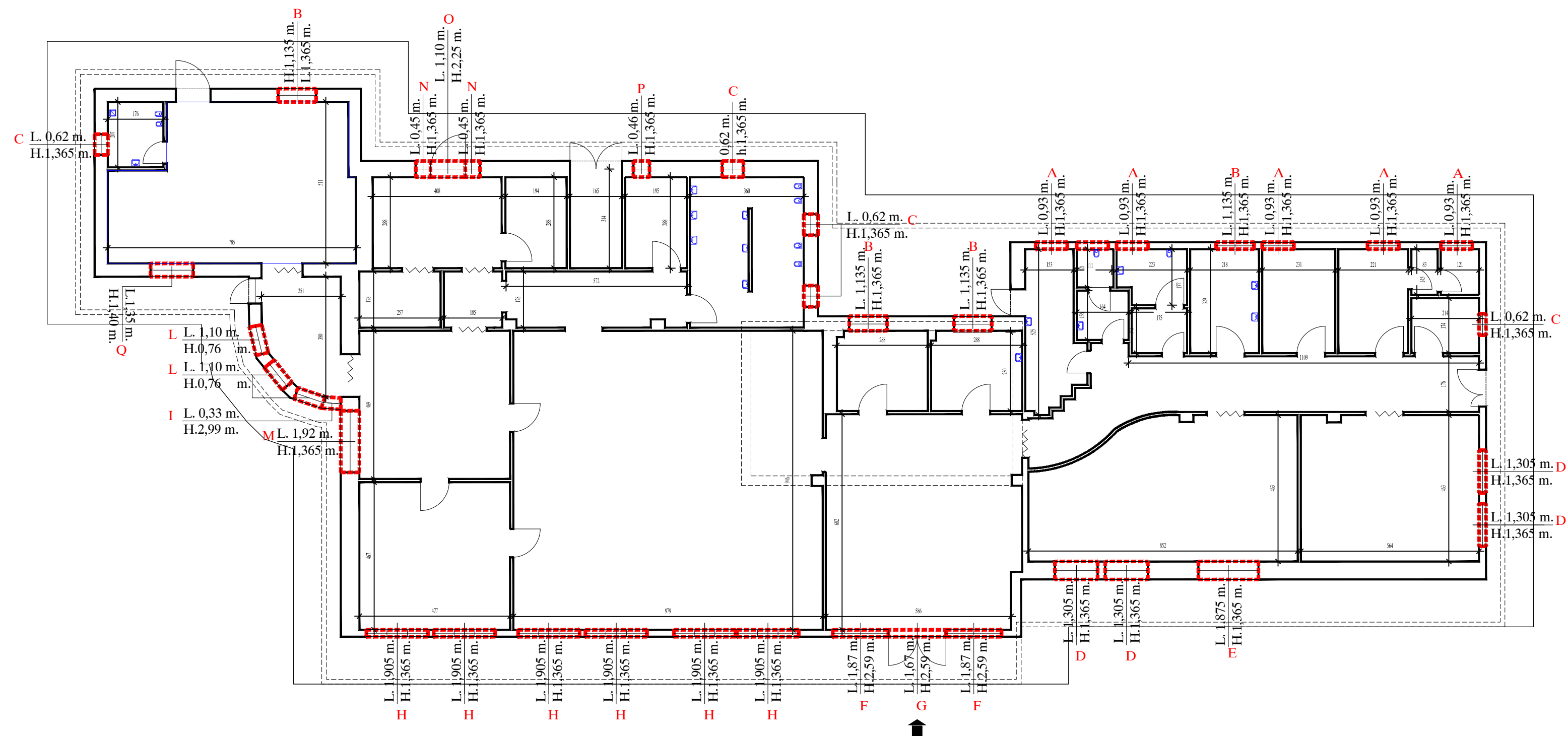
PIANTA PIANO TERRA ASILO NIDO PETER PAN
