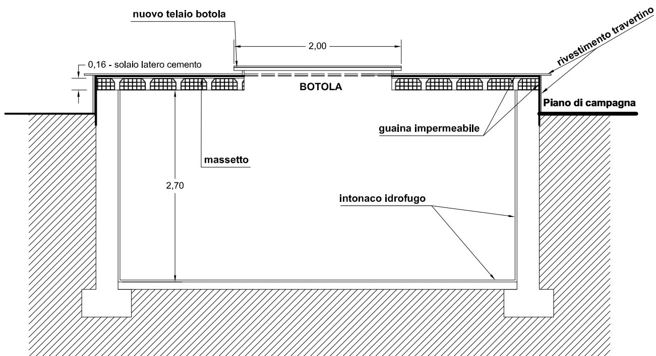
Sezione A-A' - Ossario
