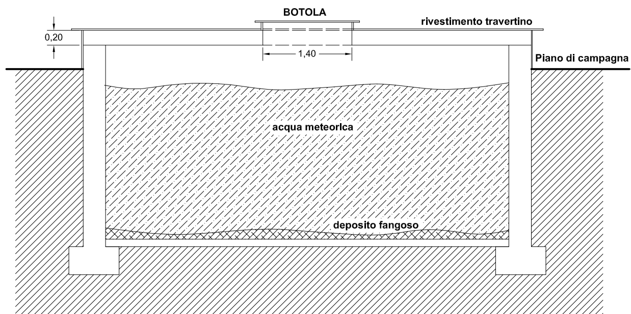
Sezione A-A' - Ossario
