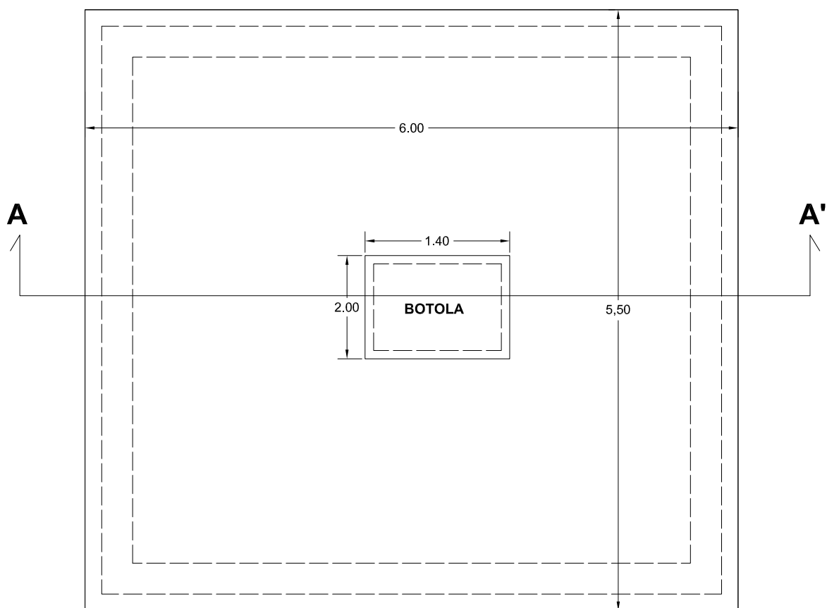
Pianta Ossario
