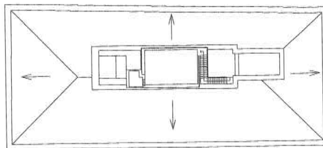
Palazzo Comunale Planimetria copertura
